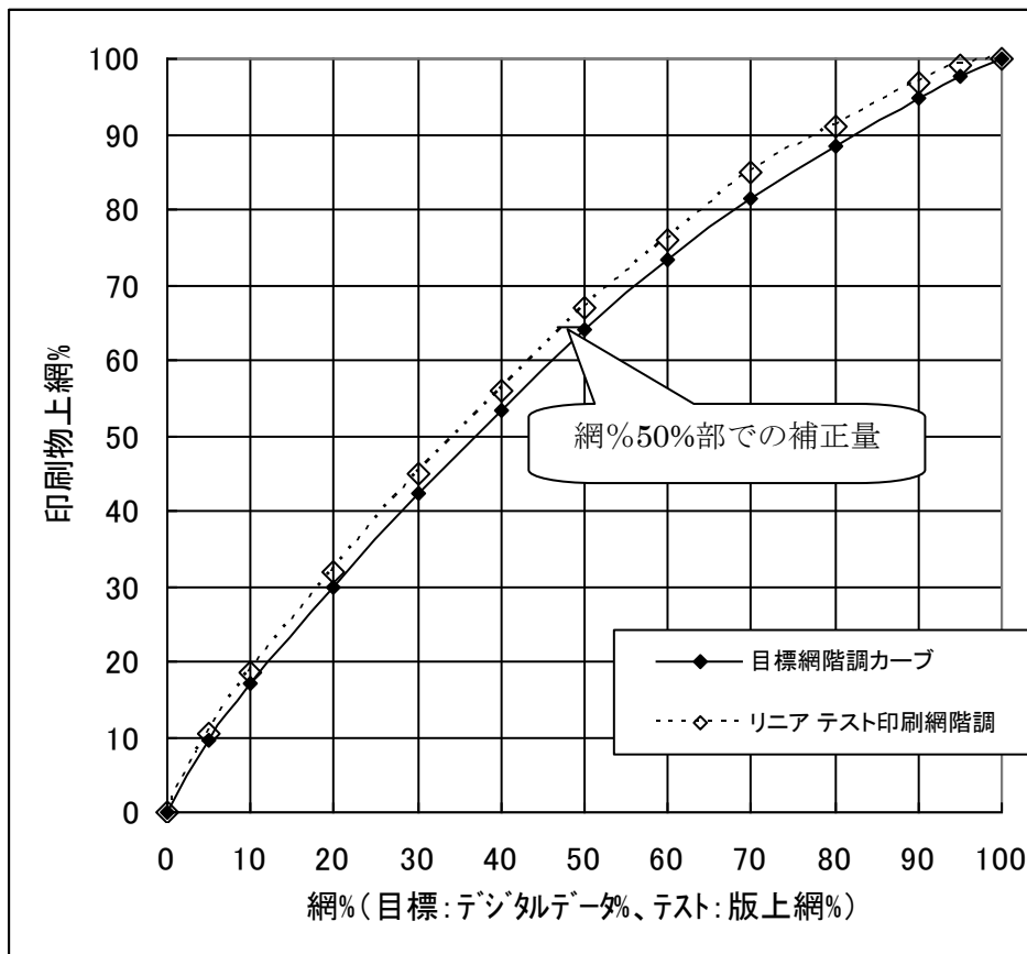
図表 5-4 網階調カーブのグラフ
